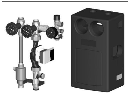
Afb. 1.1 Overdrachtstation DN25
