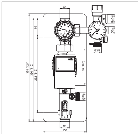
Afb. 4.1 Pompgroep, 130 (180) mm DN 25
