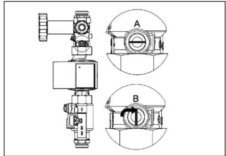
Afb. 6.12 Sperafsluiter (retourkogelkraan)
